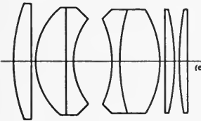
FIG. 5a. Planar f/4 . FIG. 5b. Biotar f/1.4 . FIG. 5c. Xenon f/1.3 .
